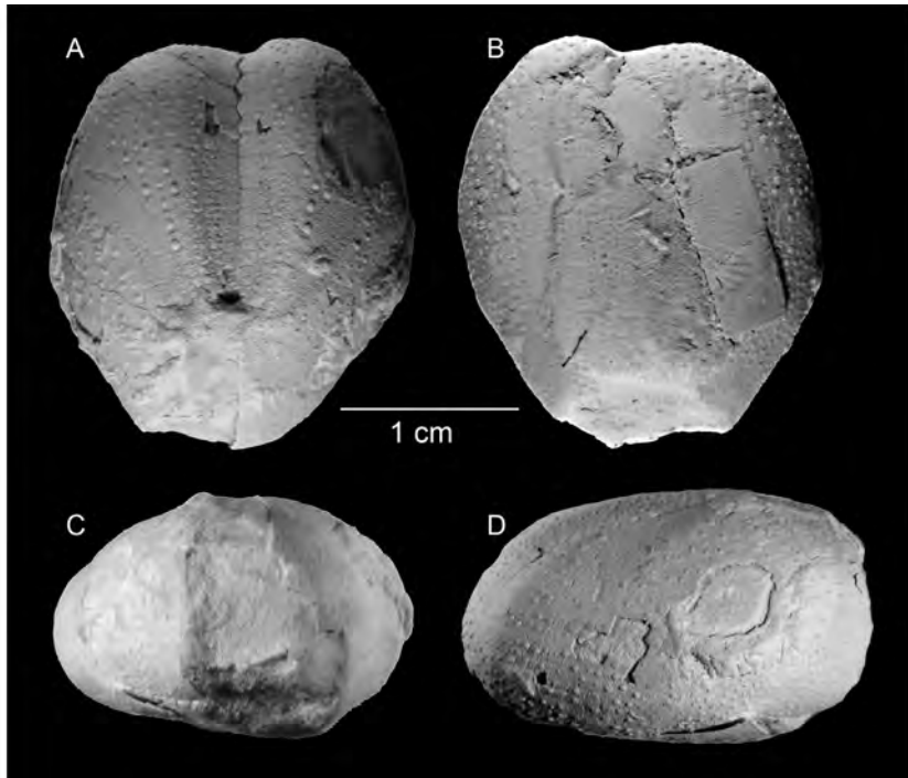
Fig. 12. Washitaster longisulcus (Adkins & Winton, 1920). IGM 2279 (Cerro de Muleros, Albiano superior). A, vista aboral; B, vista oral; C, vista posterior; D, vista lateral.
