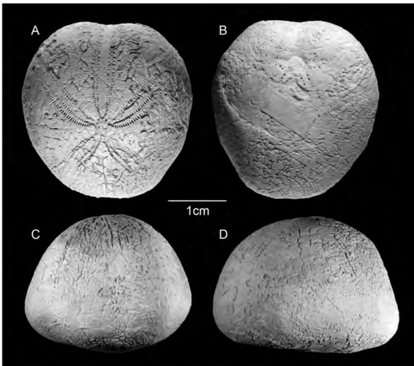
Fig. 3. Heteraster aguilerai Buitrón, 1970. Holotipo IGM 2227 (Formación San Juan Raya, Aptiano).
