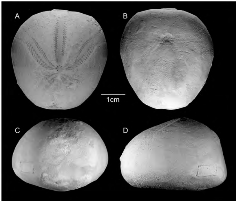
Fig 4. Heteraster alencasterae Buitrón, 1970. Holotipo IGM 2228 (Formación San Juan Raya, Aptiano). A, vista aboral; B, vista oral; C, vista posterior; D, vista lateral.
