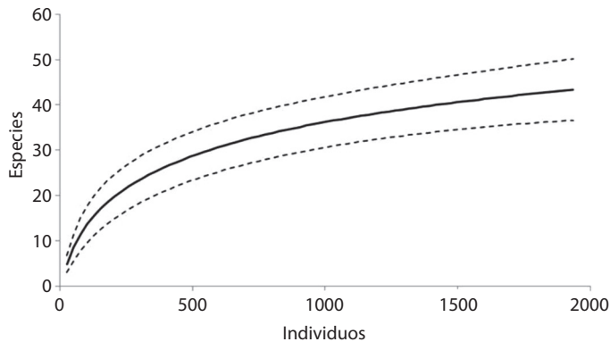
Fig. 1. Curva general de especies acumuladas durante el presente estudio. Líneas discontinuas representan los intervalos de confianza al 95 %.
